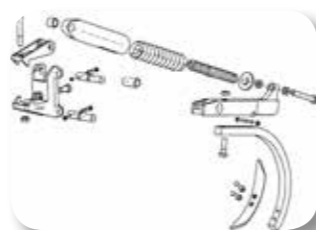
Brazo y amarre CHM
